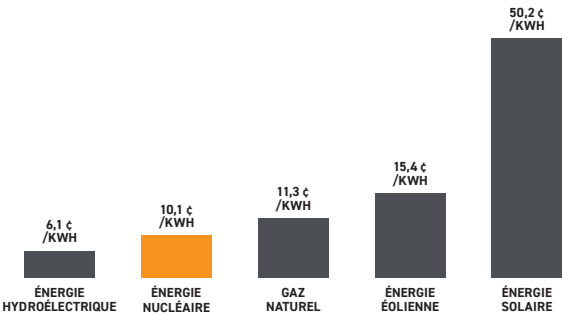
COÛT DE L'ÉNERGIE SELON LA SOURCE EN ONTARIO EN 2022
